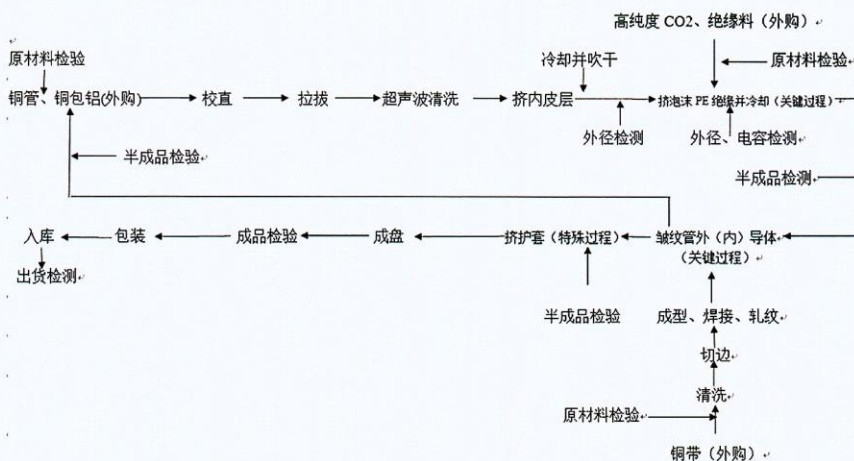
图1 馈线产品生产工艺流程图
