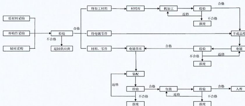
图1 馈线附件产品生产工艺流程图
