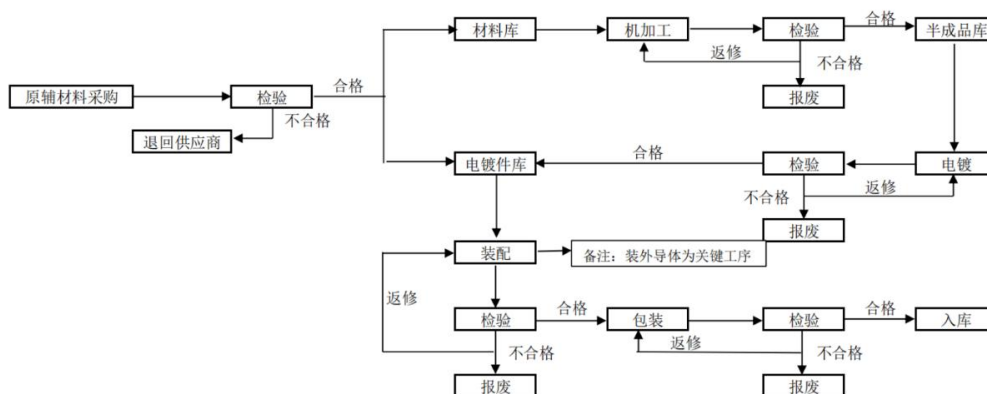
图 2 产品生产工艺流程
